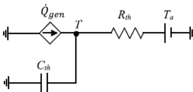
شکل ۱۰: مدل حرارتی
