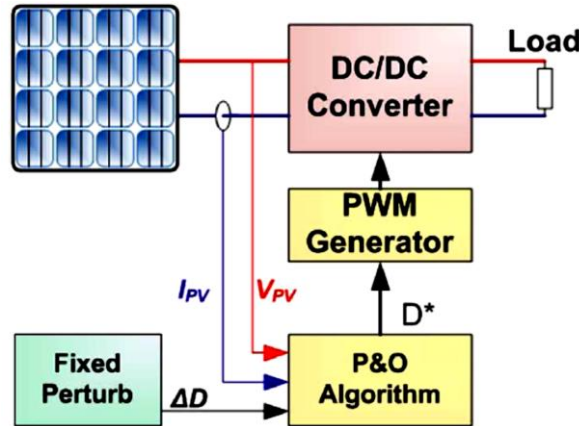
شکل ۱۸: طرح کلی روش تعدیل یافته‌ی P&O
