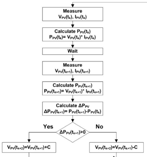
شکل ۱۶: فلوچارت روش P&O
