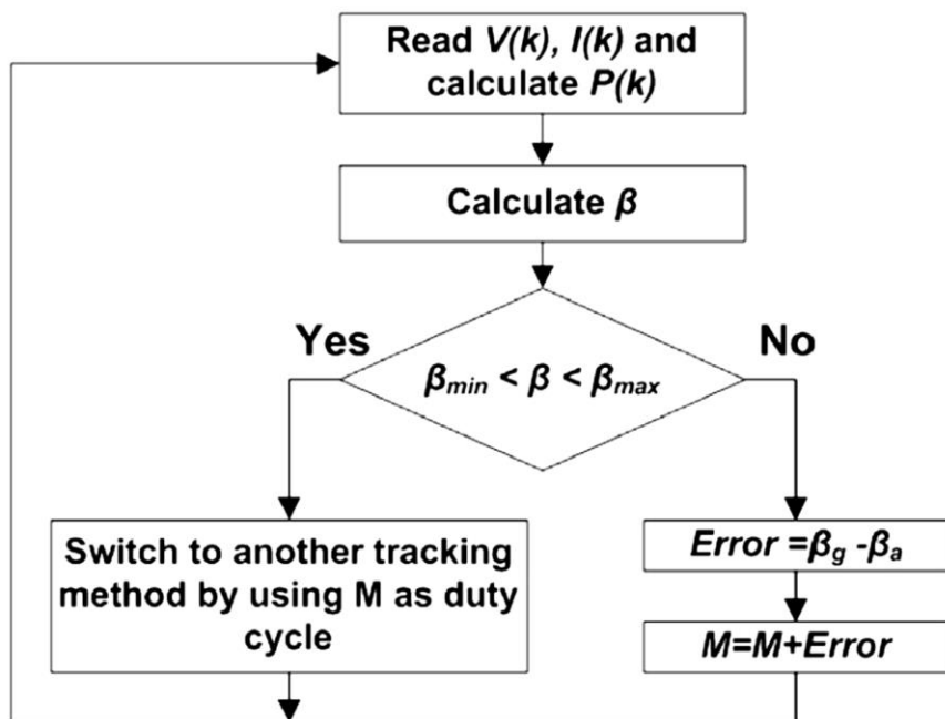
شکل ۲۵: فلوچارت روش \beta
