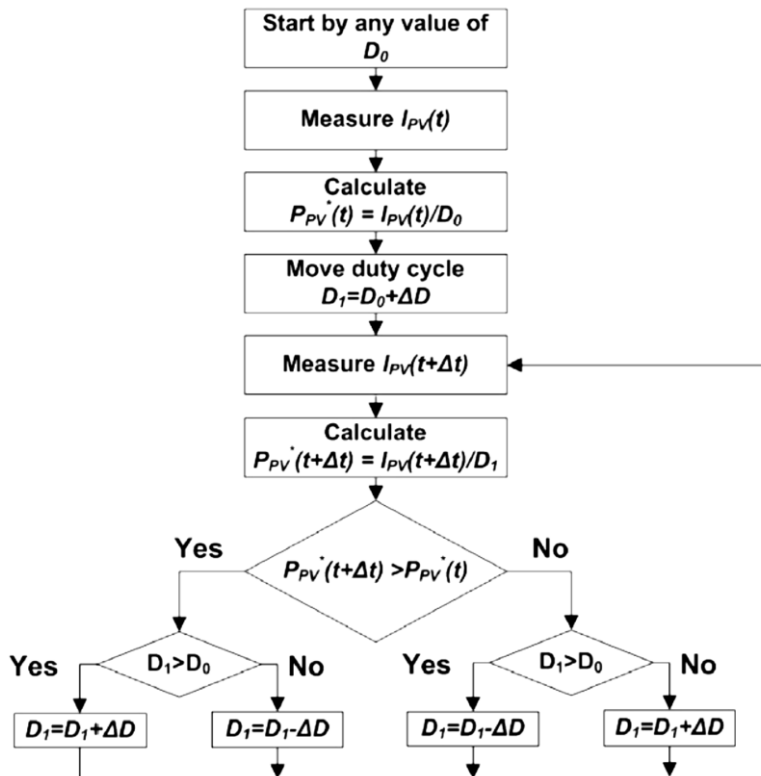
شکل ۱۳: فلوجارت روش سلول PV
