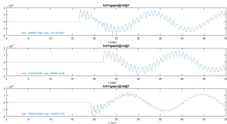
شکل ۲۰: نمایش شکل موج TRV در شبیه‌سازی شبکه معادل
